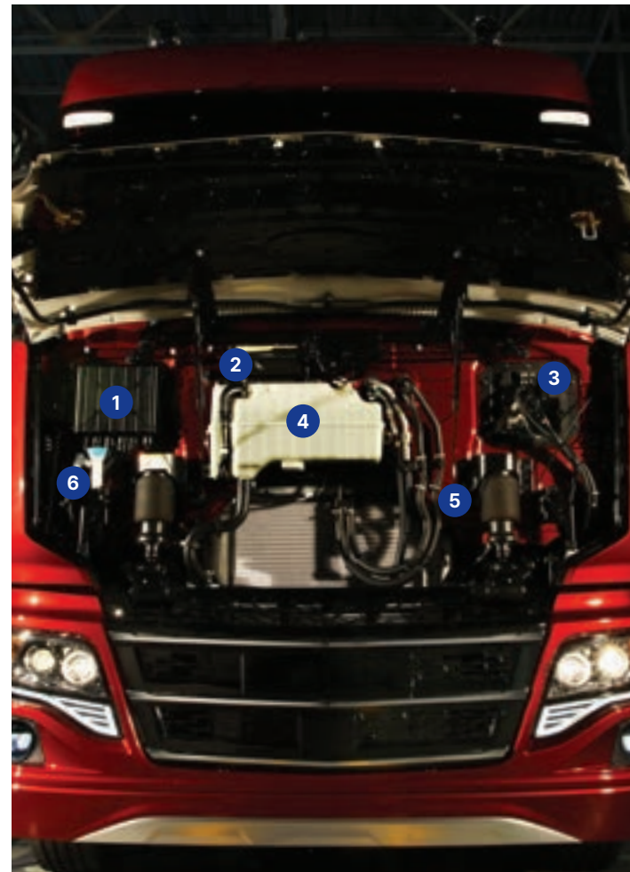
① 멀티 커넥터 ③ 브레이크 페달 모듈 ⑤ 전방 캡 서스펜션 ② 에어컨 필터 ④ 냉각수 탱크 (서지탱크) ⑥ 워셔액 주입구
